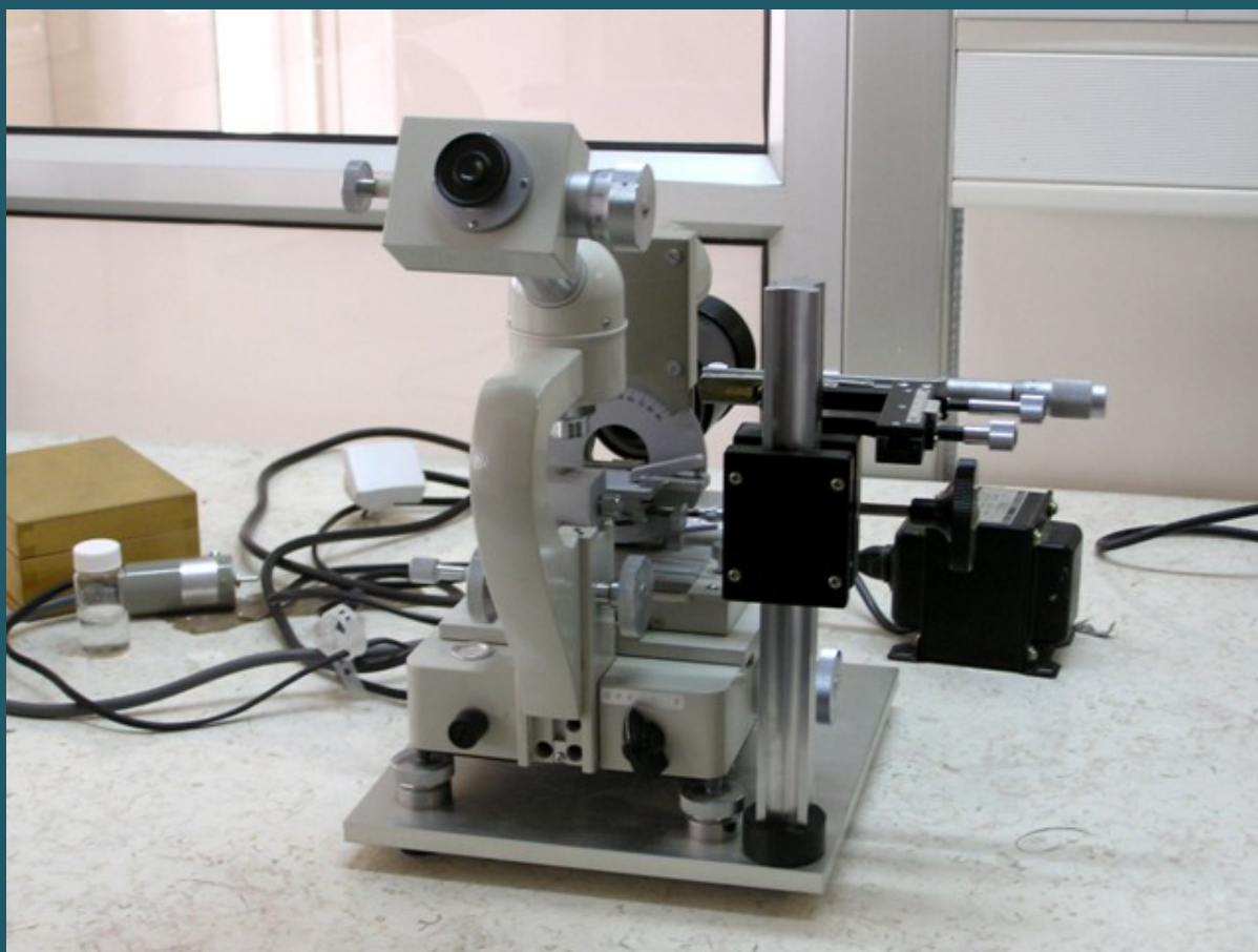
Прибор для измерения угла смачивания
