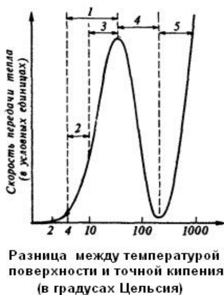
Рис.2 Кривая кипения воды. 1 – пузырьчатое кипение, 2 – изолированные пузырьки, 3 – столбы и «куски» пара, 4 – переходный режим кипения, 5 – пленочное кипение.
