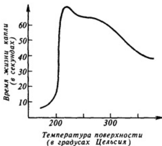
Рис.3 Кривая времени жизни капли воды на горячей поверхности.
