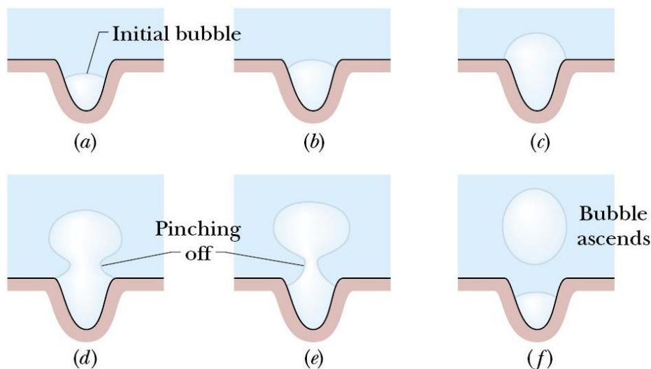
Рис.1 Образование пузырьков. (a) – пузырек газа, который удерживается на неровностях поверхности сосуда, (b)-(f) – пузырек растет, отрывается и поднимается.
