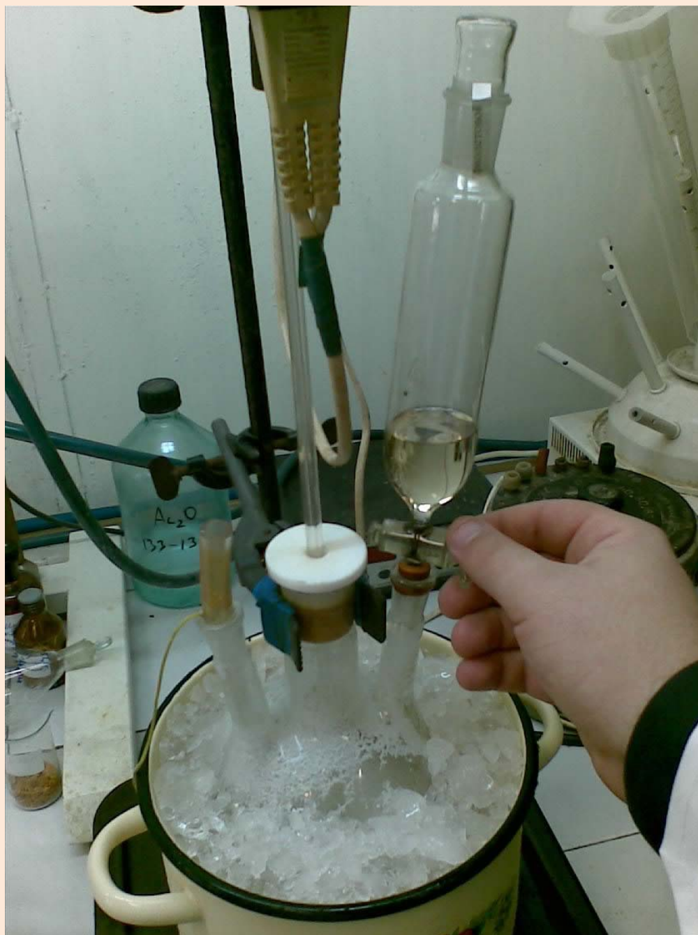
Добавление хлористого тионила к аспартату в абсолютном этаноле
