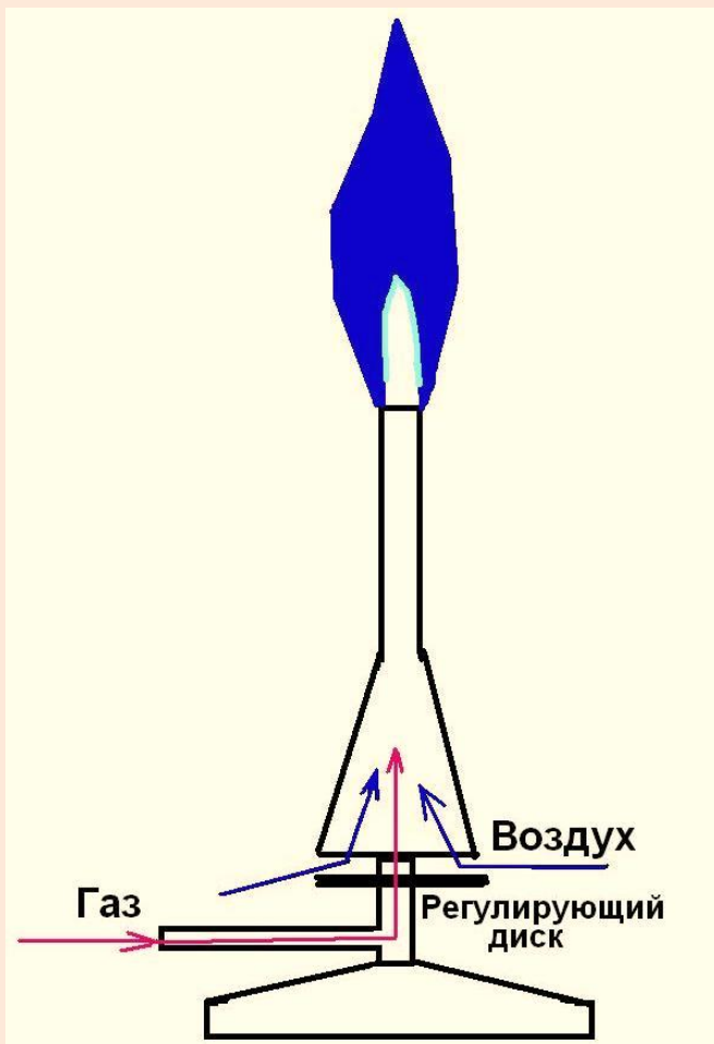
Схема Горелки Теклю.
