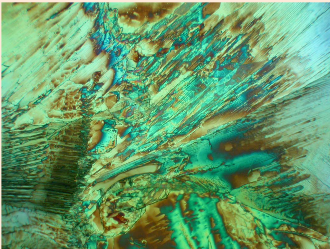
Пикриновая кислота (поляризационный микроскоп)
