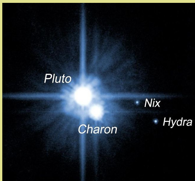
Плутон и три его известных спутника. Плутон и Харон — два ярких объекта в центре, правее — два слабых пятнышка — это Никта и Гидра
