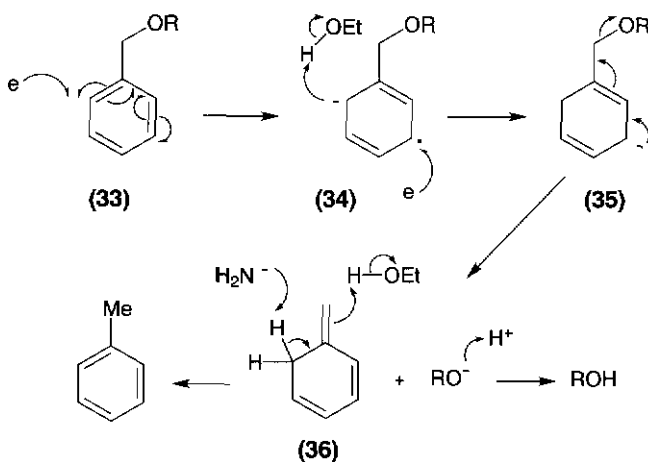
Scheme 12.11.
