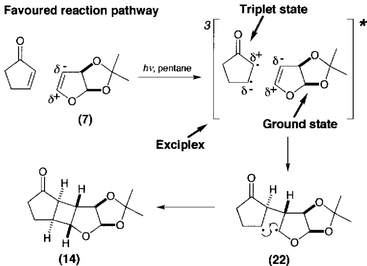
Scheme 6.7.
