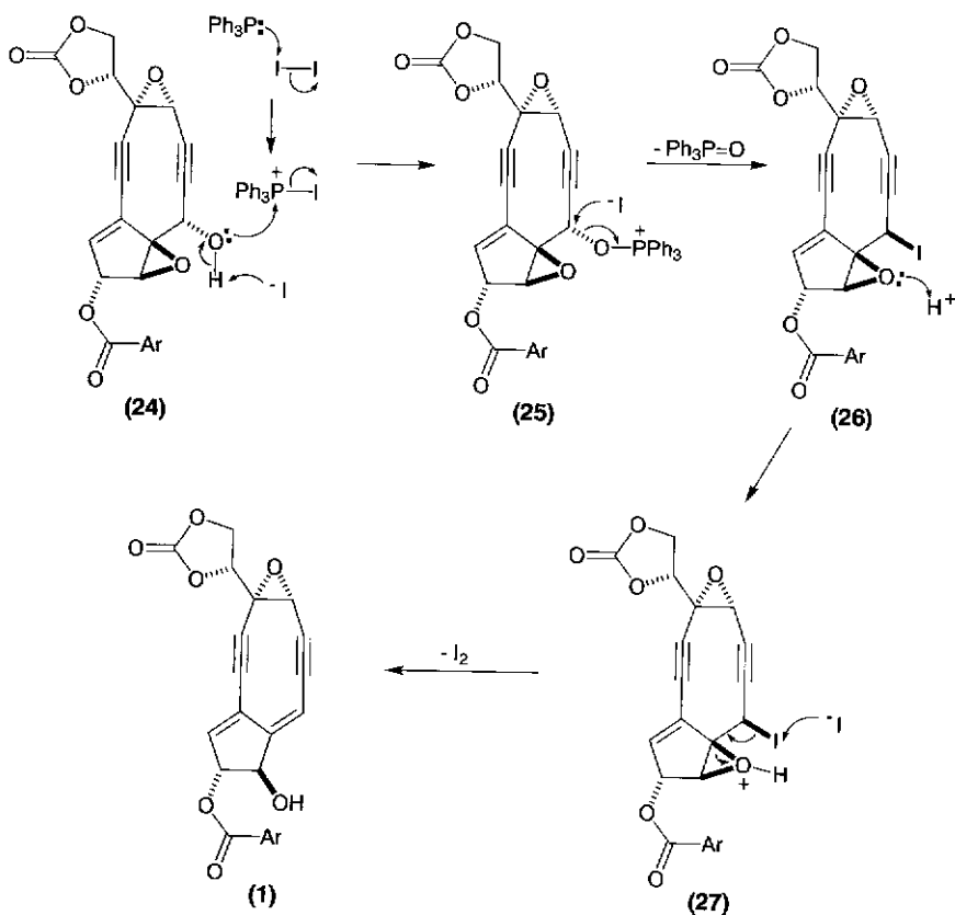
Scheme 8.12.
