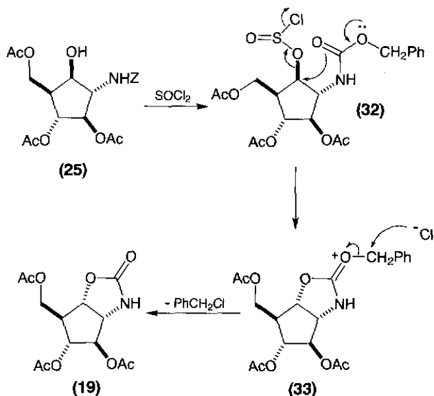
Scheme 11.11.
