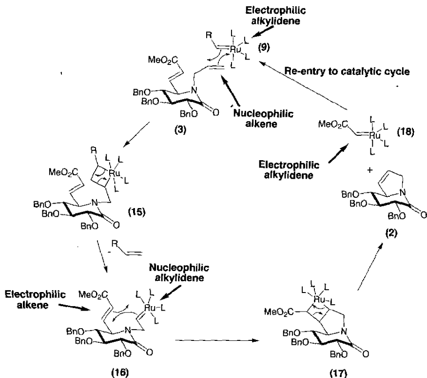
Scheme 9.4.
