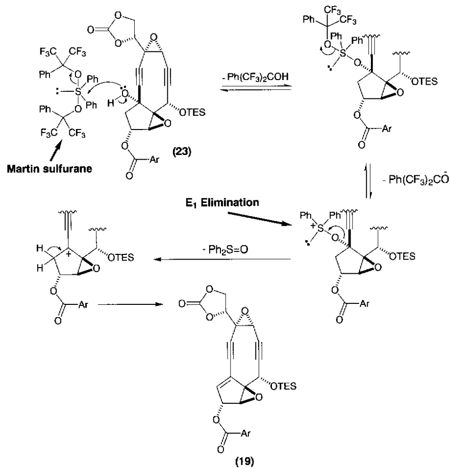
Scheme 8.11.
