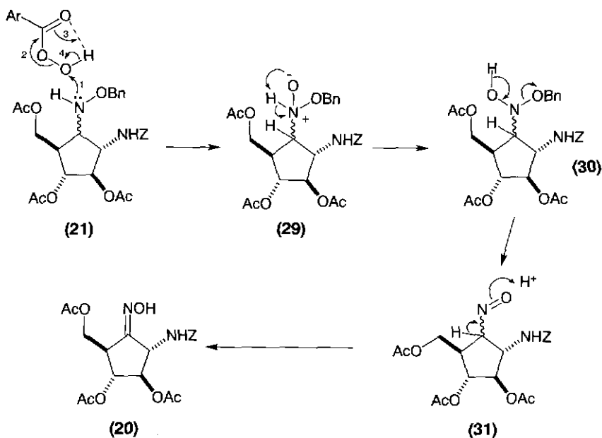
Scheme 11.10.
