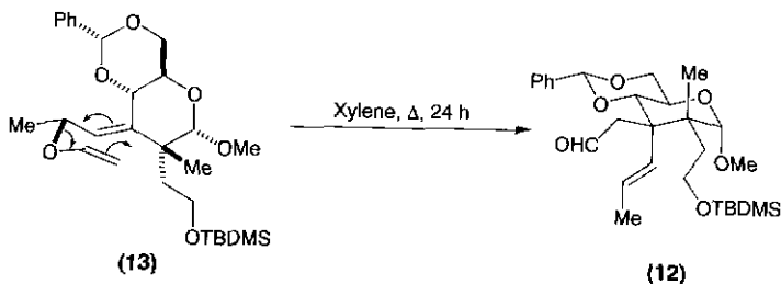
Scheme 10.7.
