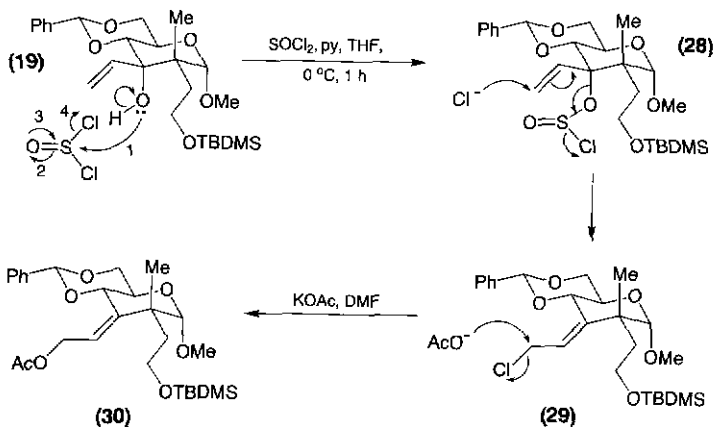
Scheme 10.6.
