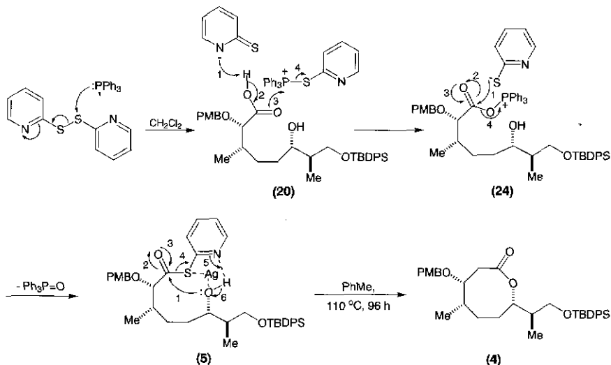
Scheme 13.5.
