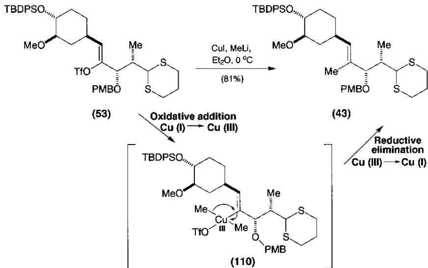
Scheme 17.30.
