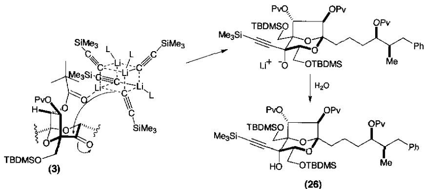
Scheme 7.10.
