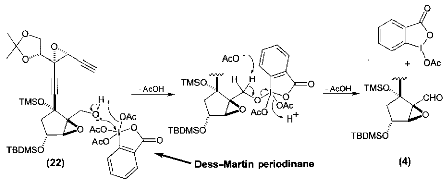
Scheme 8.10.
