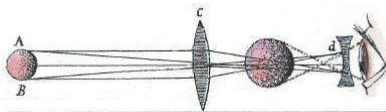
Телескоп Галилея
