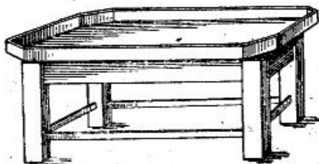
Рис. 1. Стирочный стол
