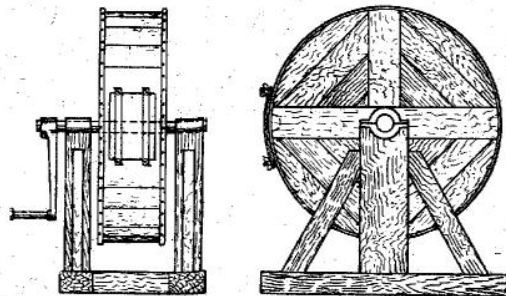
Рис. 5. Бочка для измельчения веществ.
