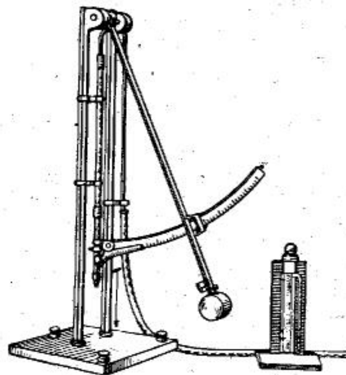
Рис. 7. Прибор для определения воспламеняемости состава
