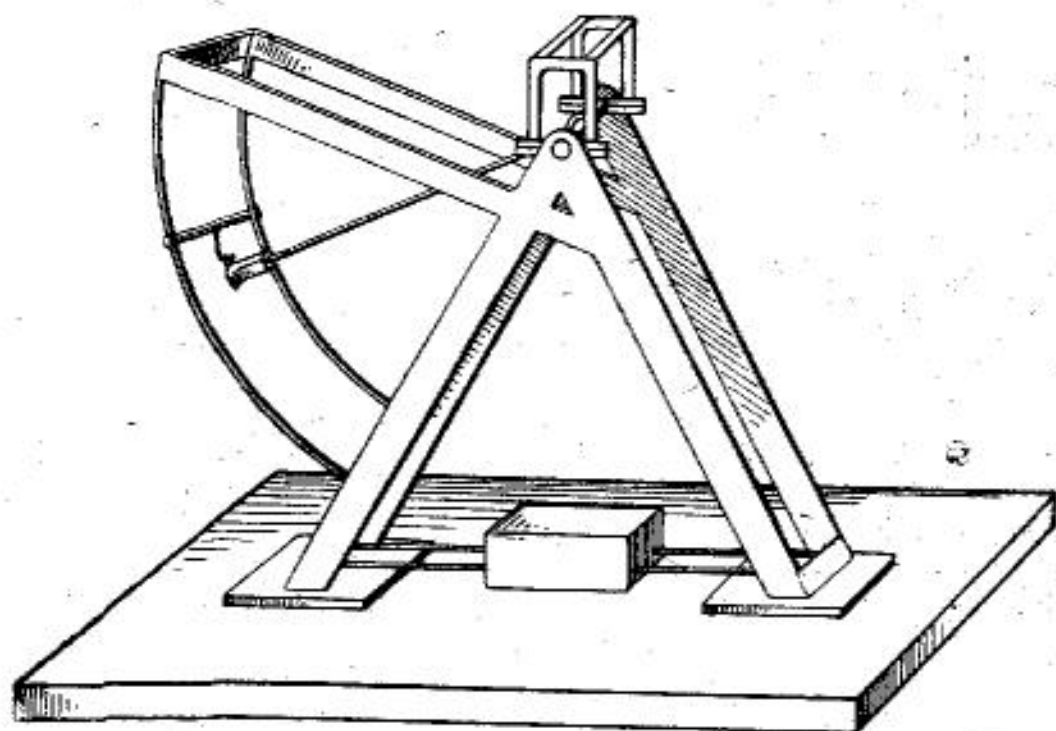
Рис. 6. Маятниковый прибор для испытания на трение
