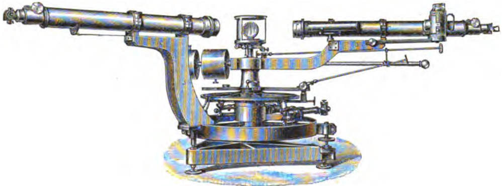
Спектрометръ астрофизической обсерваторіи въ Потсдамѣ. (Съ фотографіи.)
