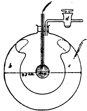
Расположеніе опыта для полученія искусственныхъ лучей короны. (По Пюпяну.)
