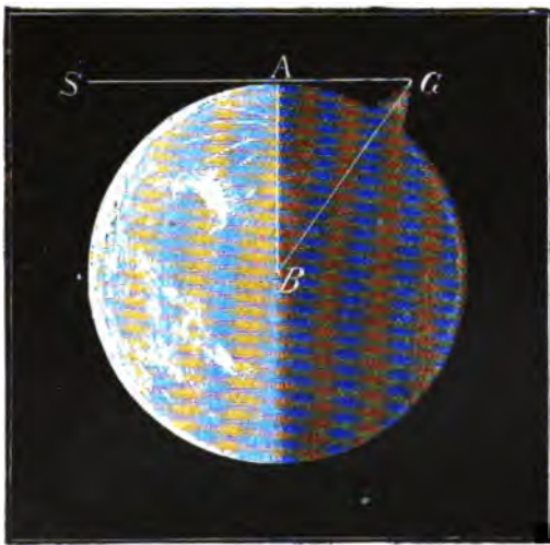
Опредѣленіе высоты лунной горы.
