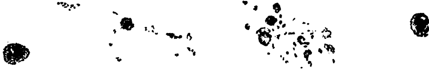
Солнечныя пятна: рядъ пятенъ, слѣдовавшихъ за большимъ февральскимъ пятномъ 1892 г., по рис. миссъ Э. Броунъ 17 февраля. См. стр. 287.
