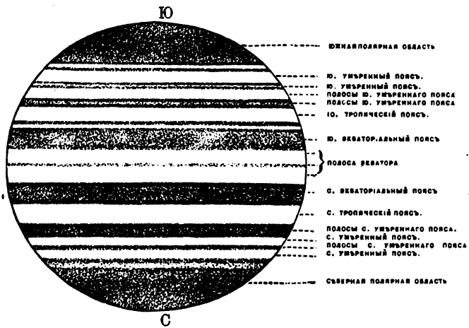
Схематическое изображение поясовъ на Юпитерѣ.
