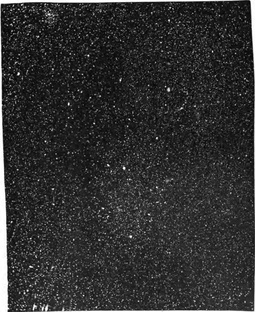
Фотографія одного участка Млечнаго Пути вблизи звѣзды \epsilon въ Лебедѣ. Получена Бернеромъ 25 сент. 1890 г. при экспозиціи въ 5 часовъ 20 мин.
