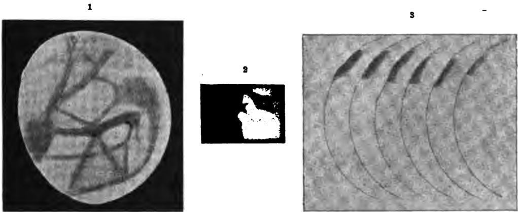
Линія терминатора на Марсѣ: 1) выступъ, наблюдавшійся Дугласомъ 11 августа 1894 г.; 2) выступъ вблизи моря Сирень, наблюдавшійся Дугласомъ 19 августа 1894 г.; 3) выемки, наблюдавшіяся на обсерваторіи Ловеля 24 августа 1894 г.
