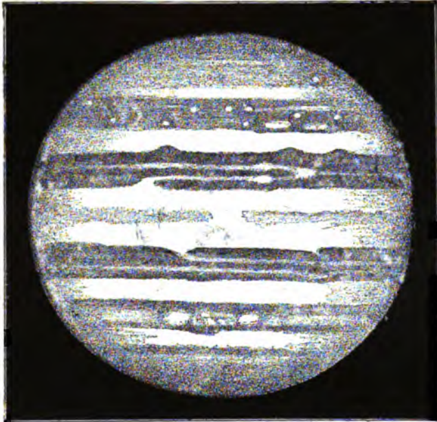
Юпитеръ Рис. Килера, на Ликской обсерваторіи 10 июля 1889 г.
