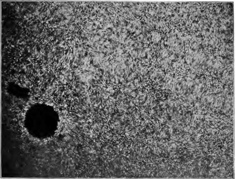
Строение грануляции на подобие ивовых листьев и симметрично образованное пятно. По фотографии 10 июня 1887 (минимум пятен).
