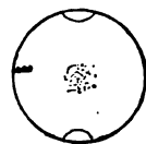
Первый извѣстный рисунокъ Марса съ полярными пятнами, Маральди (1704 г.).
