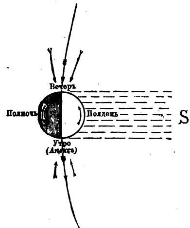
Движеніе земли сквозь рой падающихъ звѣздъ.
