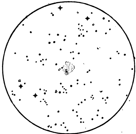
Новая звѣзда (n) въ Орионѣ 1895 г. съ окрестными звѣздами. По А. Риккѣ. a, b, c неподвижныя звѣзды созв. Ориона.
