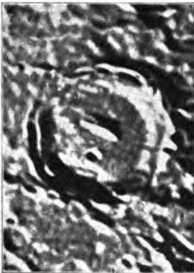
Лунный кратер Арзахель: 1) 15 августа 1888; 2) 27 августа 1888. Рисовано по 10-кратному увеличенію оригинальнаго негатива Ликской обсерваторіи Л. Вейнекомъ въ Прагѣ.
