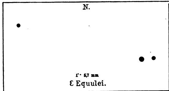
Тройная звѣзда \varepsilon Equulei.
