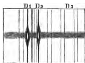
Линія D въ спектрѣ солнечнаго пятна: измѣненія линій поглощенія надъ солнечнымъ пятномъ.
