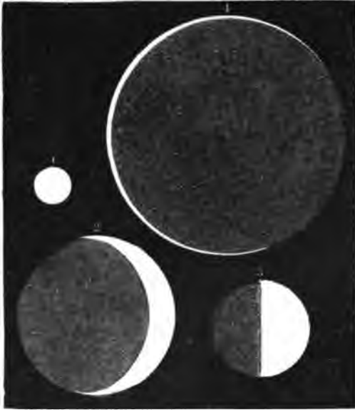
Фазы и размѣненія относительной величины Венеры: 1) въ верхнемъ соединеніи, 2) въ первой четверти, 3) въ периодъ наибольшаго блеска, 4) вскорѣ послѣ нижняго соединенія, съ далеко выступающими рогами серпа. Рис. Варнарда 1890 г.
