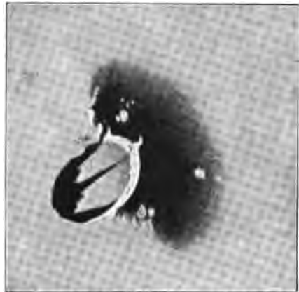
Циркъ Платонъ при восходѣ солнца. Рис. Л. Вейнека въ Прагѣ, 10 ноября 1884.
