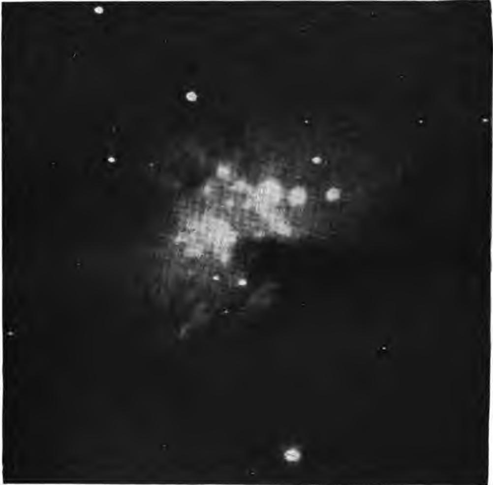
Туманность Ориона, по фотографіи Дрепера, полученной въ 1862 г. См. стр. 347.
