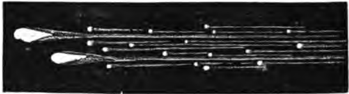
Метеоръ, наблюдавшійся 19 октября 1863 г. Шмидтомъ въ Афинахъ.
