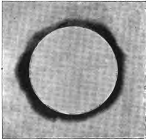
Фотографія солнечной короны; снята астрономомъ Липской обсерваторіи при полномъ солнечномъ затменіи 16 апрѣля 1893 г. въ Перу.
