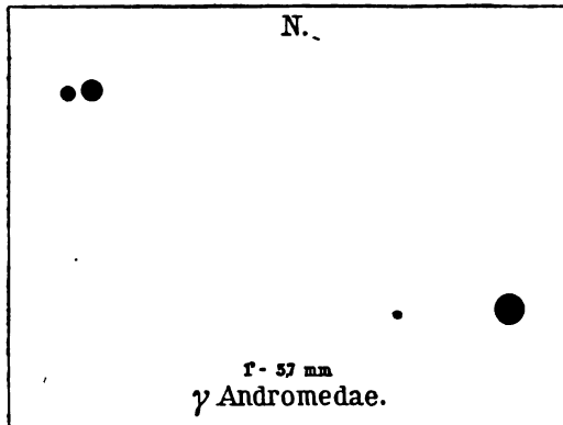
Тройная звѣзда \gamma Andromedae.
