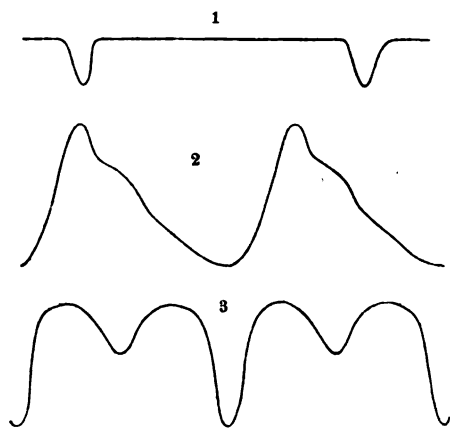
Кривыя измененія блеска переменныхъ звѣздъ: 1) Альголя, 2) \delta Cephei, 3) \beta Lyrae.
