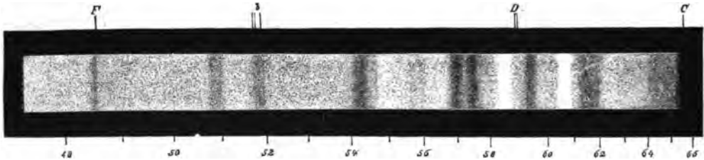
Спектръ Урана, по фотографіи Килера въ Ликской обсерваторіи.
