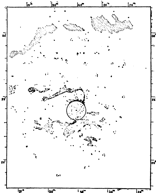
Туманныя образованія, окружающія группу Плеядъ. По фотографіи Бернерда.
