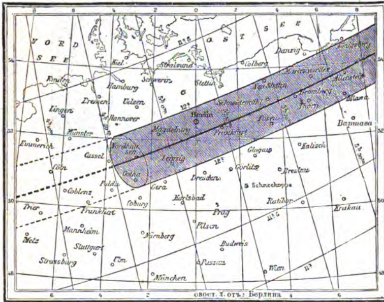
Ходъ лунной тѣни во время солнечнаго затменія 7/18 авг. 1887 г.
