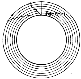
Дѣйствіе рефракціи или преломленія лучей въ атмосферѣ.
