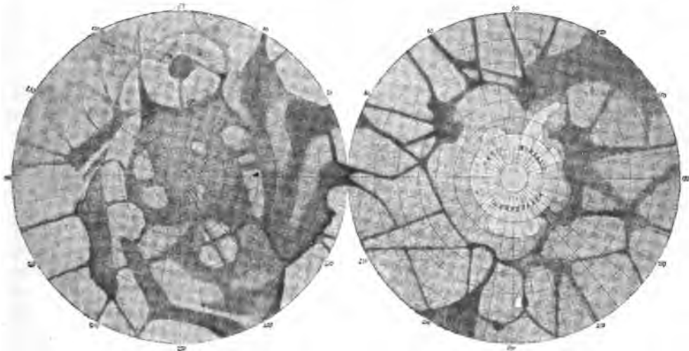
Видъ Марса съ полюсовъ во время противостоянія 1879 г., по рис. И. В. Скиапарелли.
