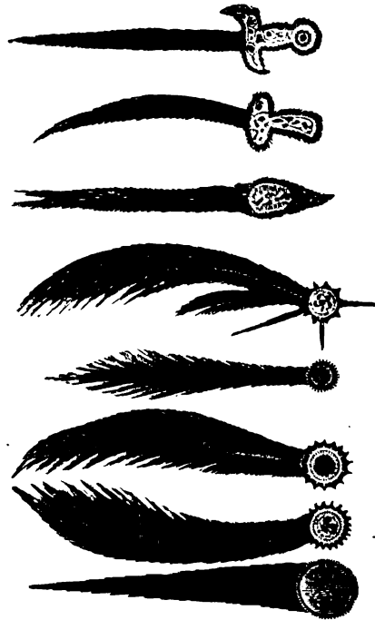
Рисунки кометъ изъ Кометографій „Гевеля“.
