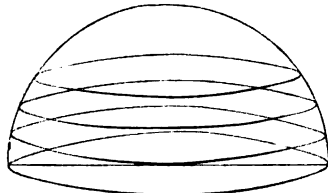
Видимые пути свѣтилъ на одномъ изъ полюсовъ земли.
