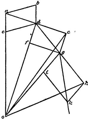
Доказательство общей применимости 2-го закона Кеплера при дѣйствіи центральныхъ силъ.
