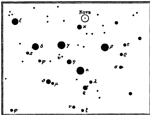
Положеніе звезды Тихо 1572 г. (Nova Cassiopeiae).
