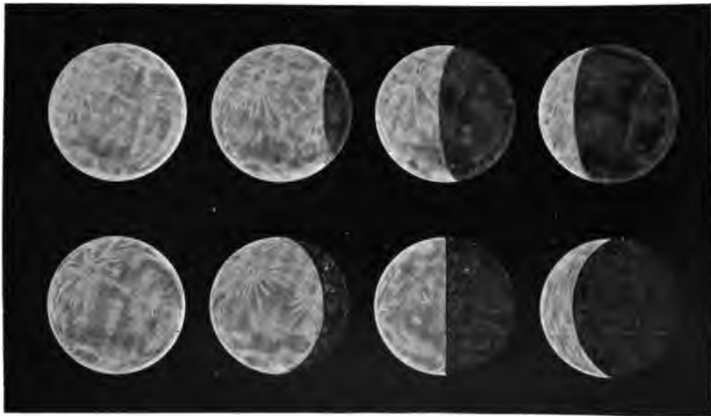
Фазы луннаго затмеія и обычныя лунныя фазы.
