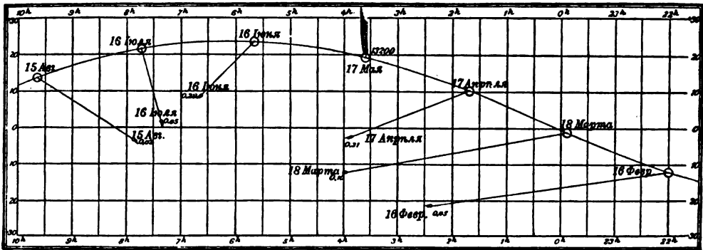
Орбита одной невидимой кометы. Маленькіе кружки указываютъ мѣсто солнца въ обозначенные рядомъ съ ними моменты времени. Во всѣхъ точкахъ положенія воображаемой кометы, соединенныхъ съ кружками прямыми линиями, указаны теоретическія величины ея яркости.
