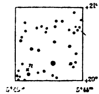
Карта, показывающая положеніе Nova Orionis. По Боннскому каталогу. См. нижній рисунокъ.
