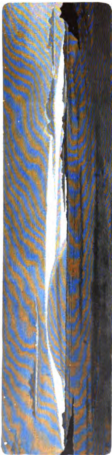
Видъ кольца Сатурна съ точки, лежащей на поверхности планеты подь 70° широты.
