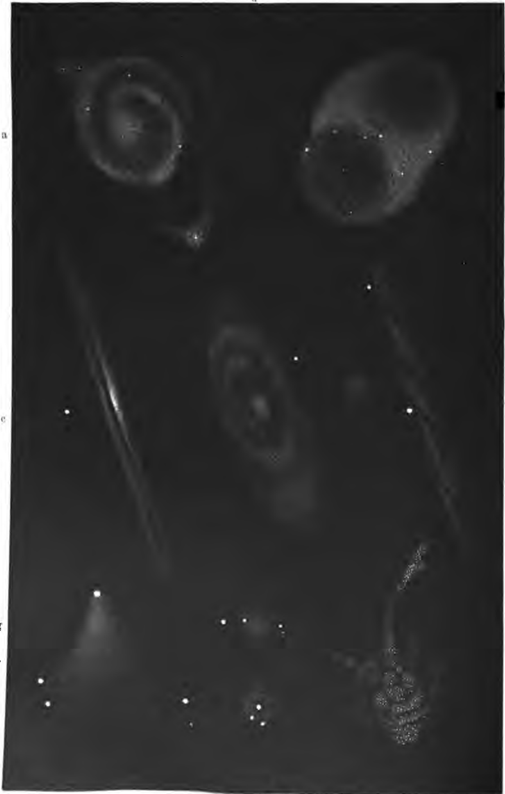
ТУМАННОСТИ РАЗЛИЧНЫХЪ ФОРМЪ.
