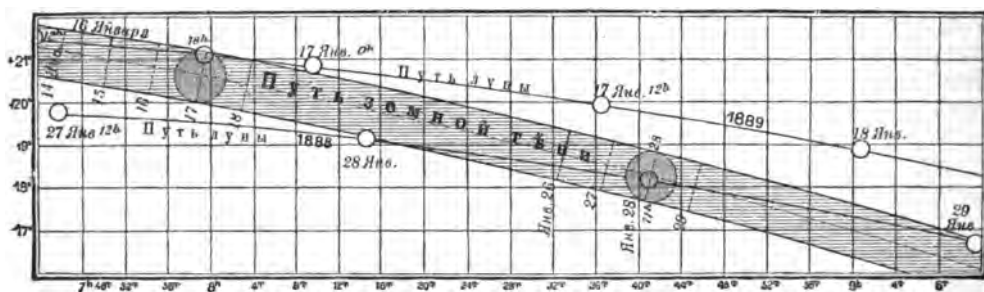
Мѣста луны и земной тѣни при двухъ лунныхъ затменіяхъ, с. стр. 534.
