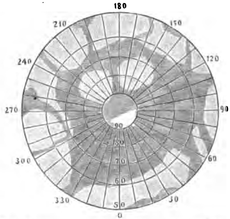
Подеженіе южнаго полярнаго пятна на Марсѣ въ 1877 г., по рис. И. В. Скиапарелли.
