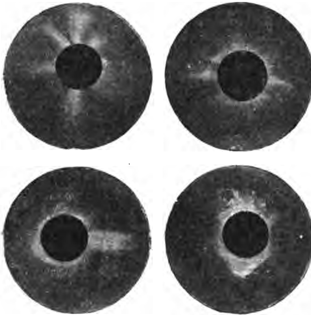
Искусственная корона, полученная Пинниомъ при помощи электрическихъ разрядовъ. Ср. текстъ, стр. 309.
