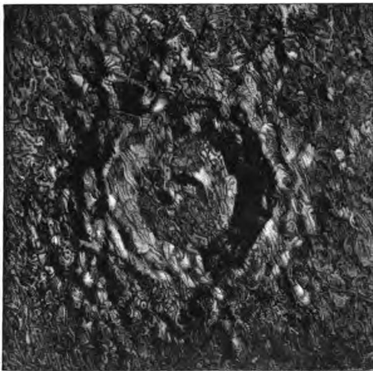
Лунный кратеръ Коперникъ, увелич. въ 14 разъ. Рис. Л. Вейнека въ Прагѣ по ориг. фотогр. Ликской обсерваторіи, 28 Іюля 1891 г.
