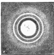
Кольца интерференціи.
