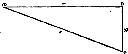
Движеніе горизонтально брошеннаго тѣла.
