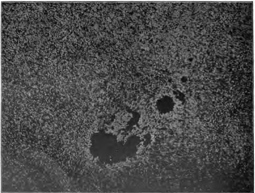
Строение грануляции на подобие рисовых зерен и группа пятен. По фотографическим снимкам Жювсена в Медон близ Парижа.
