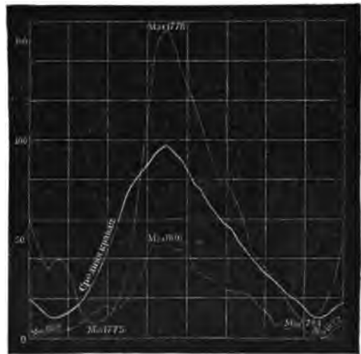
Кривая Р. Вольфа, выражающія количество солнечныхъ пятенъ.
