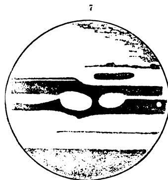
Красное пятно на Юпитерѣ: 1) 9 января 1895 г. рис., Гордона въ Патерсонѣ, Сѣв. Ам.; 2) 1880 г. рис. М. В. Мейера въ Женевѣ; 3) 20 октября 1893 г., рис. Антониади на обсерваторіи Фламмаріона въ Juvigny близъ Парижа; 4) 1889 г., рис. Килера на Ликской обсерваторіи; 5) съ полосой облаковъ, рис. 1886 г. Юнга; 6) 5 сентября 1888 г., рис. по увеличенію въ 630 разъ въ большой рефракторъ Ликской обсерваторіи; 7) 1878 г., рис. Нистена въ Брюсселѣ.
