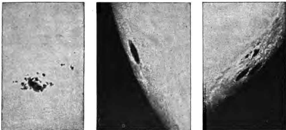
Солнечное пятно, наблюдавшееся въ августѣ 1894.
