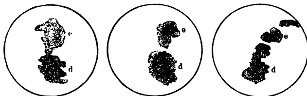
Рисунки Марса по Шрётеру, съ предполагаемыми движущимися облаками.
