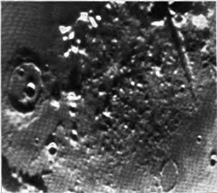
Часть лунных Альп с большою поперечною долиною.
