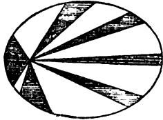
Эллипсъ Кеплера. (Заштрихованныя площади все равны между собою.)
