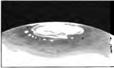
Свѣтлая точка вблизи южнаго полярнаго пятна на Марсѣ; рис. Грина 8 сентября 1877 г.
