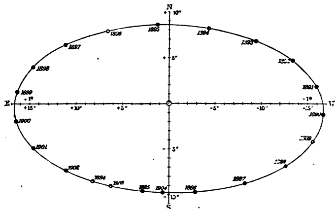
Видимыя измѣненія мѣста звѣзды \alpha Ориона вслѣдствіе нутаціи отъ 1 января 1884 до 1 января 1904 г. (покамо того ея мѣсто мѣняется еще только отъ прецессіи).
