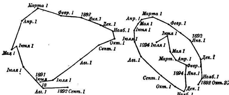
Колебанія высоты полюса въ періодъ отъ 1891 до 1894 гг.
