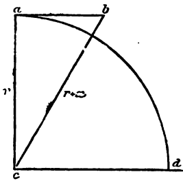
Поднятіе горизонтально брошеннаго тѣла надъ поверхностью земли.
