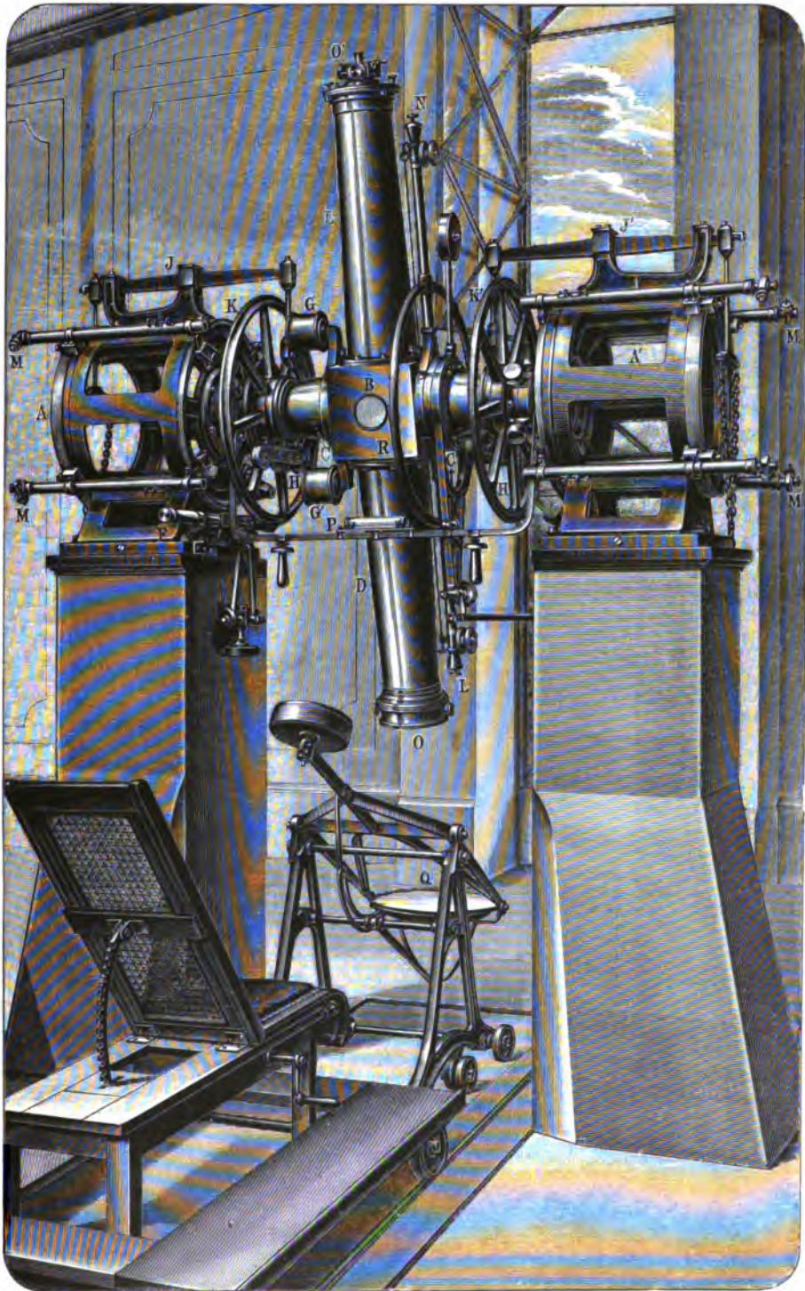
МЕРИДИАННЫЙ КРУГЪ СТРАСБУРГСКОЙ ОБСЕРВАТОРИИ.
