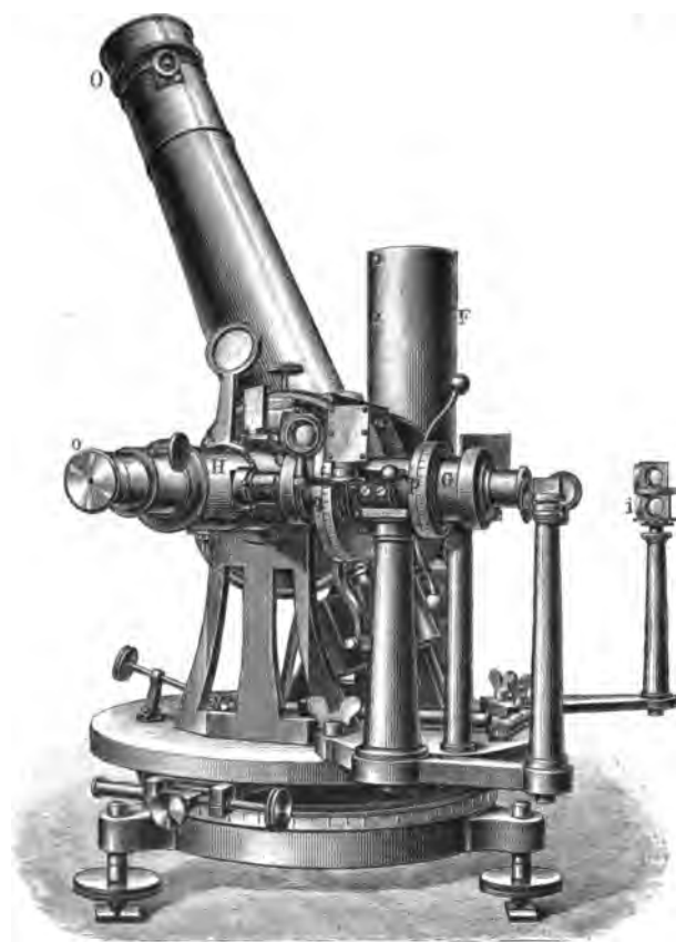
Астрофотометръ Цельнера въ Астрофизической обсерватори въ Потсдамѣ. (Съ фотографіи.)
