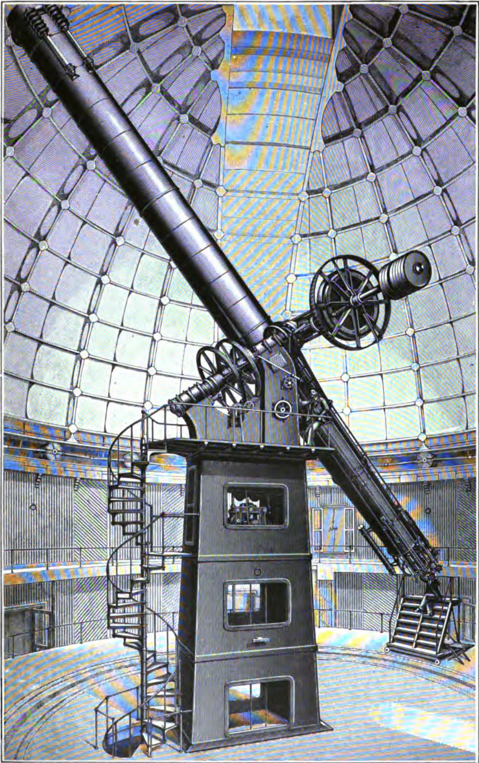
Большой рефрактор 36-ти дюймового отверстия и 15 метр. фокусного расстояния на Ликской обсерватории (гора Гамильтонъ) въ Калифорнии.
