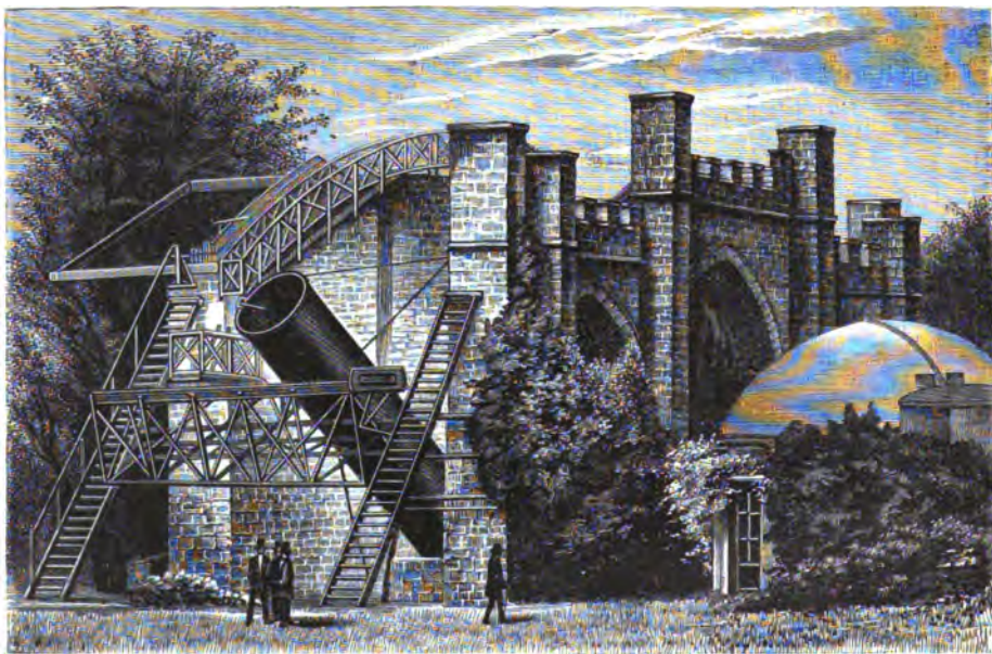
Телескопъ Левлаанъ лорда Росса въ Виррѣ-Кестлѣ, подлѣ Парсонстоуна (Ирландія).
