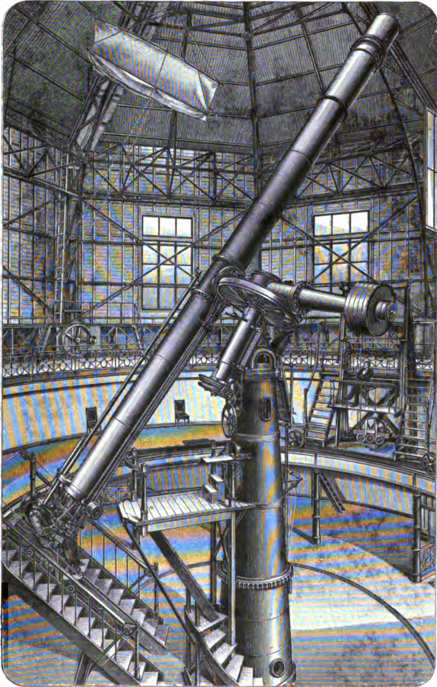
ЭКВАТОРИАЛЬ СЪ ОТВЕРСТИЕМЪ ВЪ 32 ДЮЙМА НА ПУЛКОВСКОЙ ОБСЕРВАТОРИИ, БЛИЗЪ С.-ПЕТЕРБУРГА.
