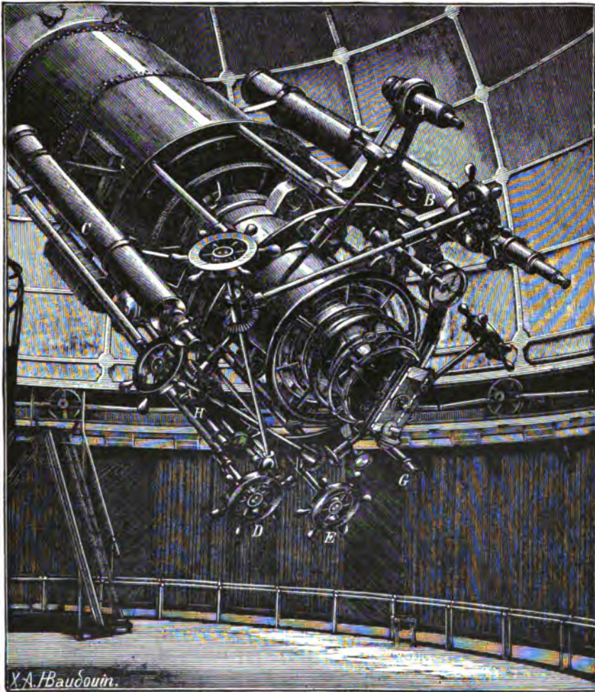
Окулярный конецъ 35-ти дюймового Ликскаго рефрактора.
