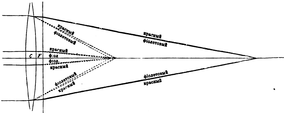
Ахроматическая комбинація стеколъ (объективъ трубы).
