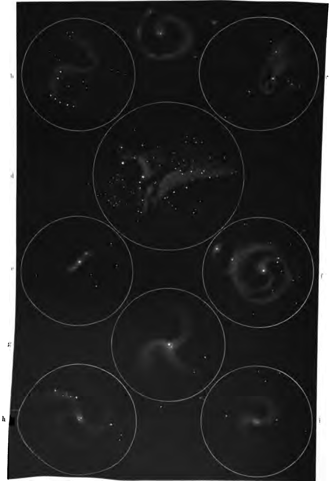
СПИРАЛЬНЫЕ ТУМАННОСТИ ПО ЛАССЕЛЮ.
