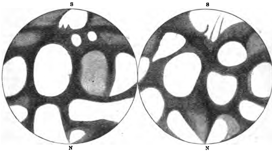
Карта Венеры, по наблюдениямъ Л. Нистена въ Брюсселѣ въ теченіи 1881—1890 гг. См. текстъ стр. 126.
