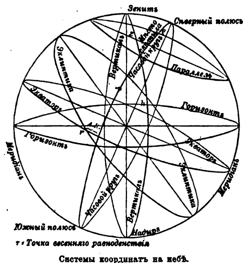
Системы координатъ на небѣ.
