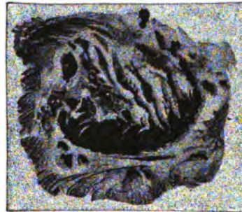
Вольшое солнечное пятно, наблюдавшееся въ февралѣ 1894 г. по рисунку Т. Морэ (Th. Mores) въ Буржѣ: 1) 20 февраля, 2) 21 февраля, 3) 22 февраля, 4) 23 февраля.
