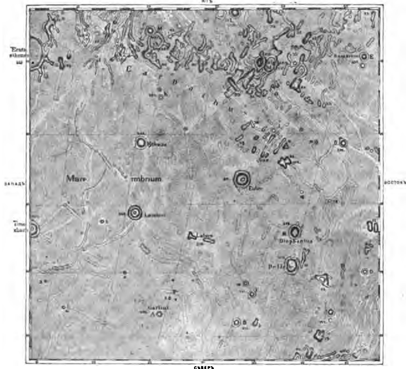
Отдѣлъ V большой лунной карты Лормана. Уменьшенная копія.
