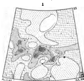
Схематическіе чертежи: 1) указываетъ мѣста одинаковой яркости въ области Млечнаго Пути, лежащей въ Лебедѣ; 2) содержатъ числа Пласмана, показывающія относительное количество звѣздъ въ той же области. Ср. текстъ, стр. 379.
