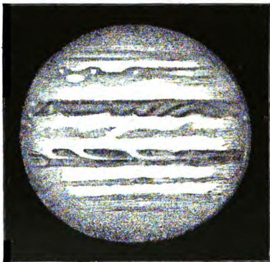
Юпитеръ. Рис. Килера на Ликской обсерваторіи 15 июля 1899 г.
