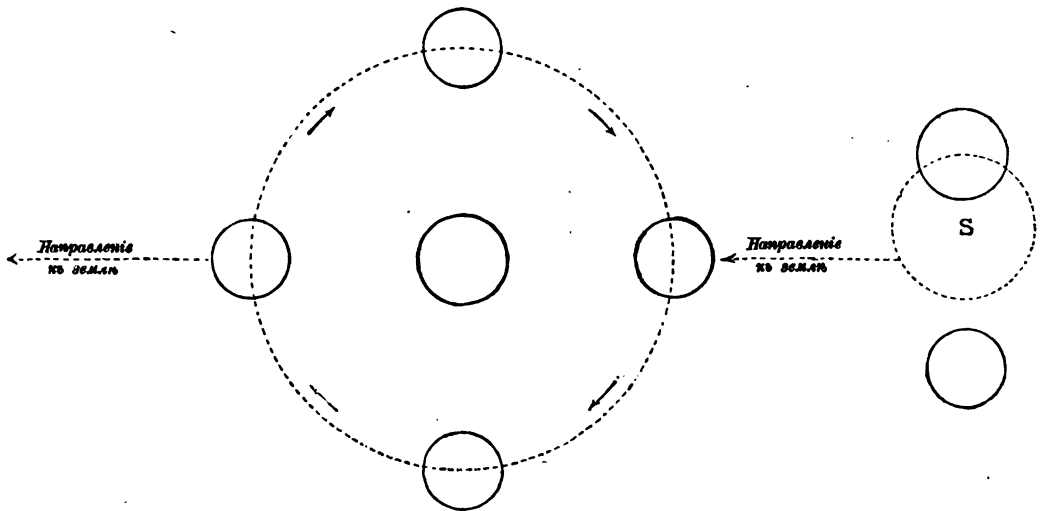
Система Альголя, по Фогелю.
