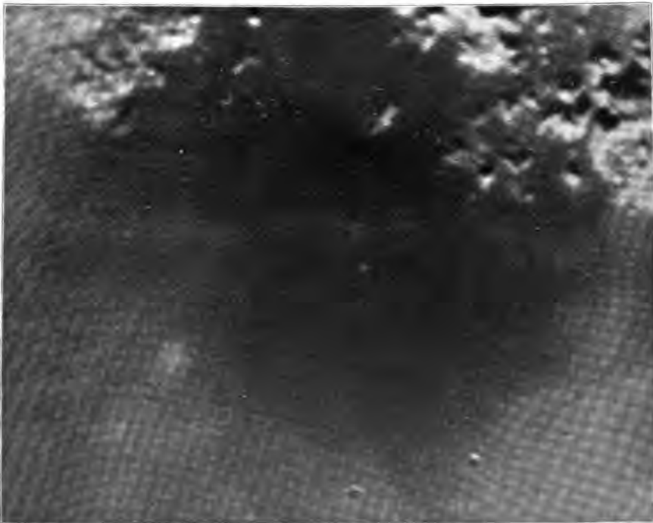
Лунный кратер Динней и его окрестности.
