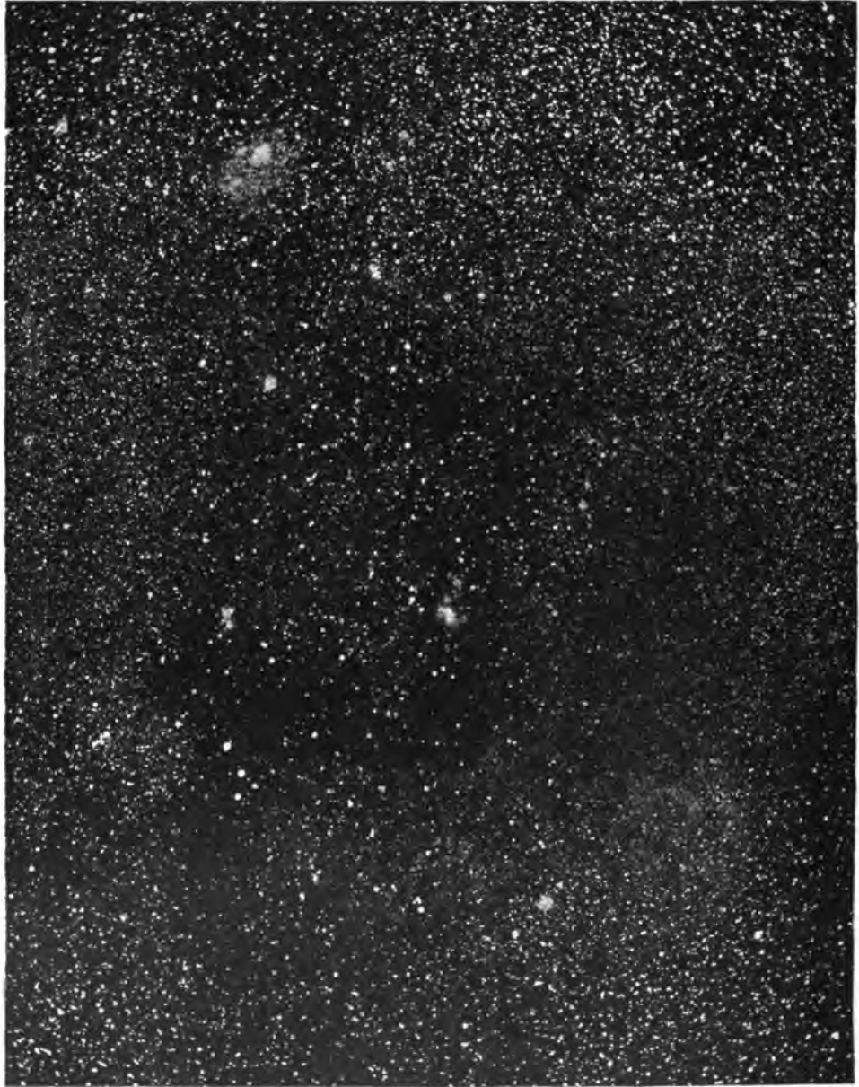
Фотографія одного участка Млечнаго Пути вблизи звѣзды 15 въ Единорогѣ. Получена Бернердомъ 1 февр. 1894 г. при трехчасовой экспозиціи.
