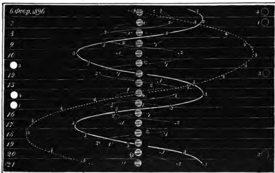
Положеніе четырехъ большхъ спутниковъ Юпитера въ періодъ отъ 6 до 21 февраля 1896 г., см. текстъ стр. 174.
