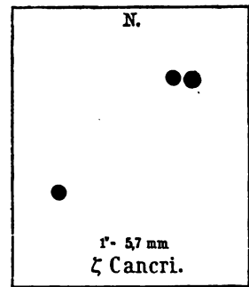
Тройная система \zeta Cancri.
