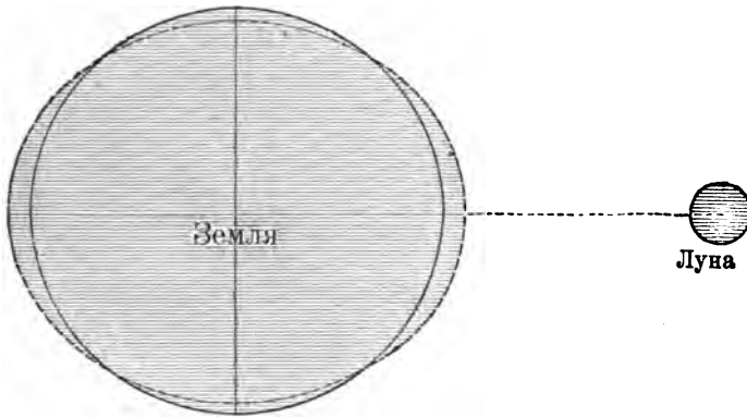
Происхожденіе приливовъ и отливовъ подъ вліаніемъ притяженія луны.
