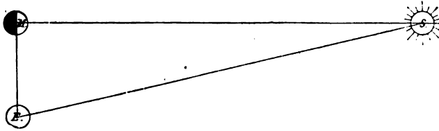
Треугольникъ: солнце — земля — луна.
