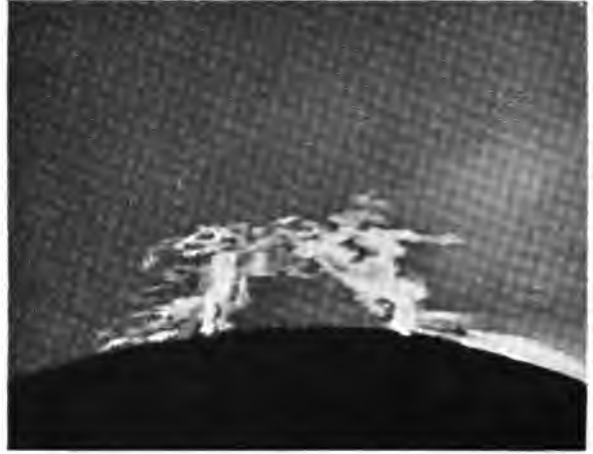
Солнечный протуберансъ, по фотографіи Георга Хэля въ Чикаго 3 июля 1894.
