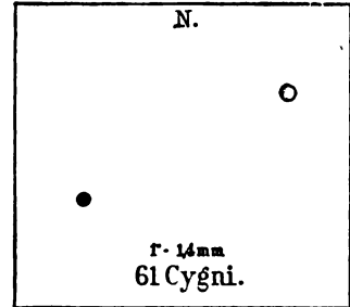
Двойная звѣзда \beta въ Лебедѣ.
