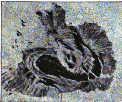
Вольшое солнечное пятно, наблюдавшееся въ февралѣ 1894 г. по рисунку Т. Морэ (Th. Mores) въ Буржѣ: 1) 20 февраля, 2) 21 февраля, 3) 22 февраля, 4) 23 февраля.
