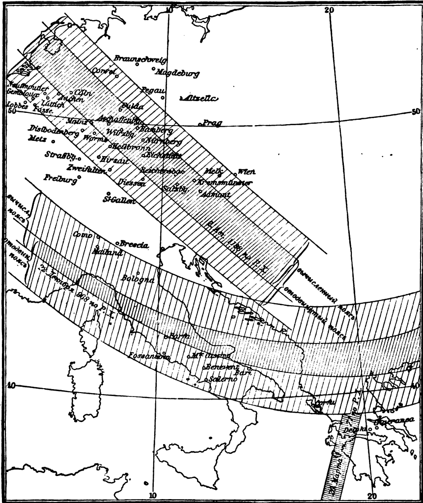
Исправленные центральныя зоны древнихъ солнечныхъ затменій.
