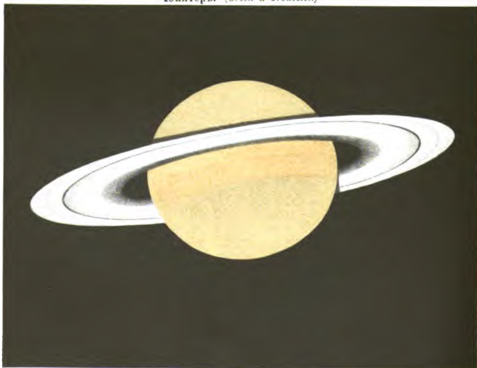
Сатурнъ. ( Barnard, Trouvelot и Mascari. )
