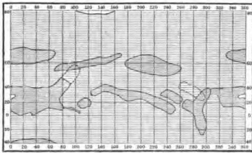
Марсъ по Вашингтонскимъ наблюденіемъ 1877 года. Фламмарионъ, „La planète Mars“.
