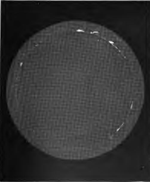
Фотографическій снимокъ хромосферы съ протуберансами, Георга Хэля въ Чикаго.
