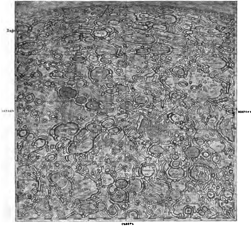
Отдѣлъ XXIII большой лунной карты Лормана. Уменьшенная копія.
