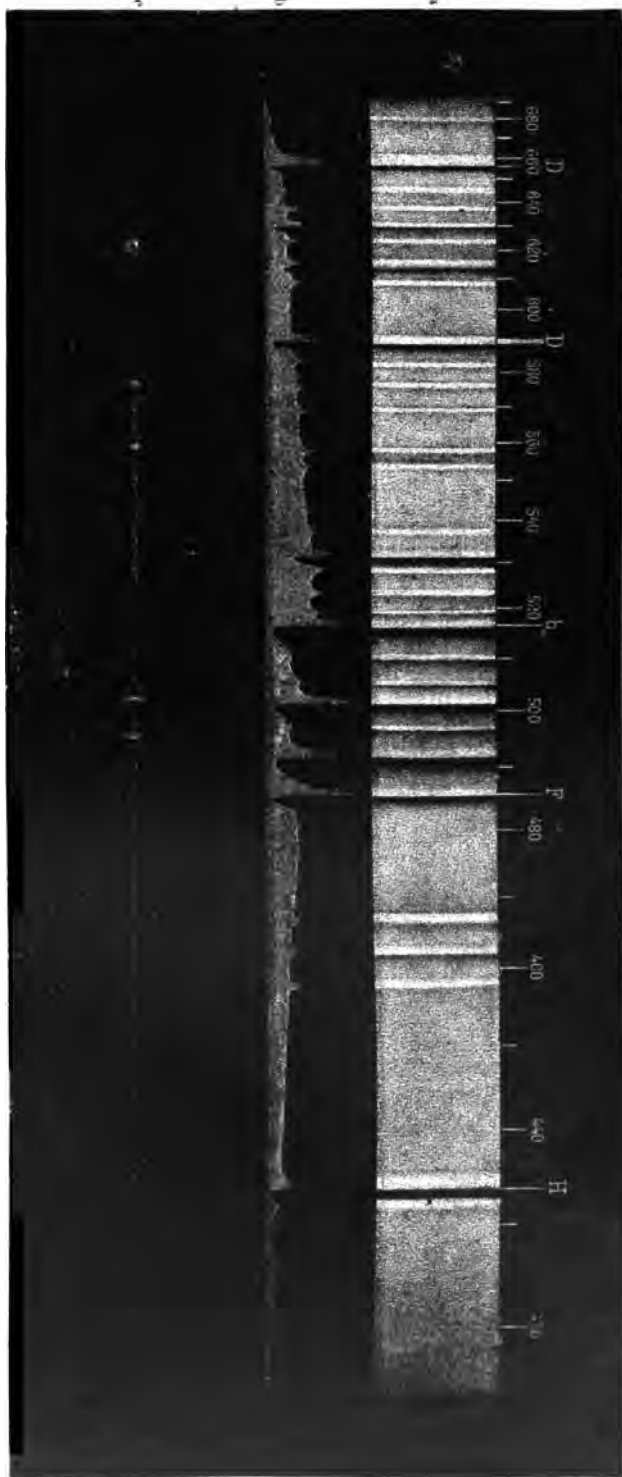
Спектры новой звѣзды въ Возничемъ: а) 23 февраля 1892 г., б) апрѣля измѣненія яркости этого спектра, в) въ августѣ 1892 г., по Кемпбеллу.
