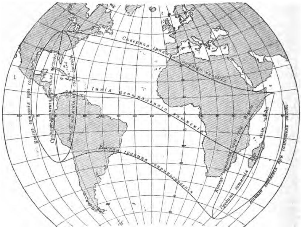
Границы солнечнаго затменія 29 авг. 1886
