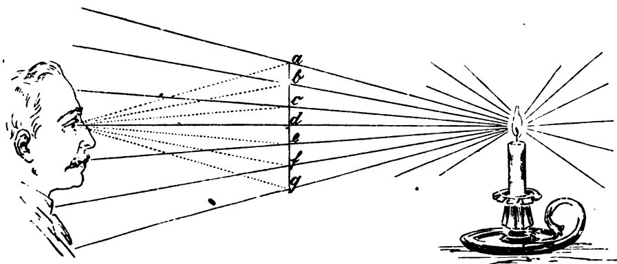
Распространеніе свѣта въ пространствѣ.
