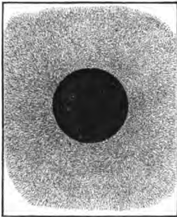
Расположеніе желѣзныхъ опилокъ вокругъ полюса магнита (линія силъ). Ср. текстъ, стр. 310.
