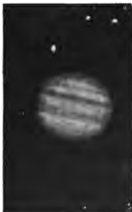
Планета Юпитеръ, фотографированная на Гарвардской обсерваторіи въ Кембриджѣ (Сѣверная Америка).
