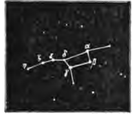
Маленькая карта, показывающая положеніе звѣзд \zeta и \epsilon Urae Majoris, какъ оно представляется невооруженному глазу. См. стр. 320.
