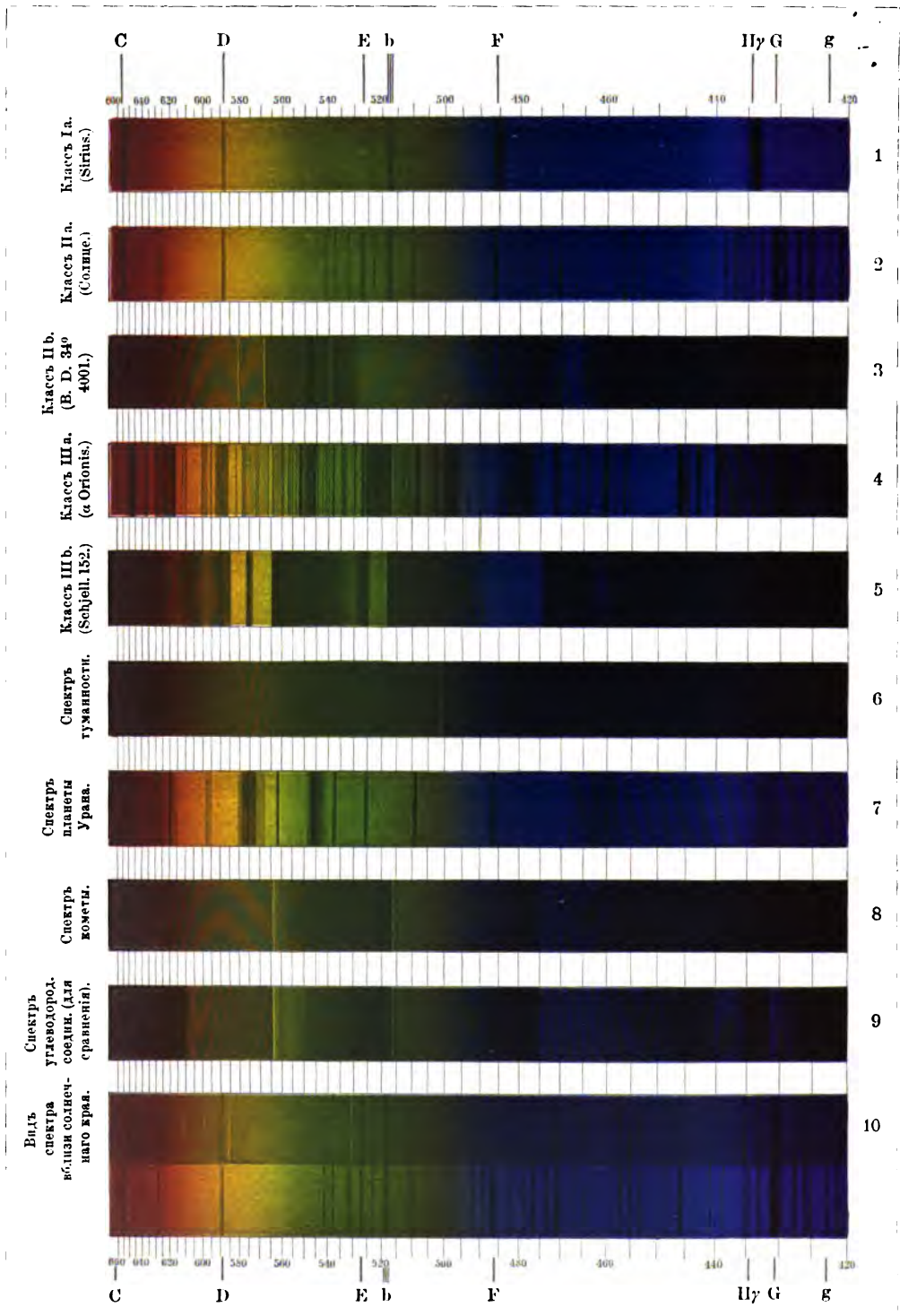
СПЕКТРЫ НЕБЕСНЫХЪ ТѢЛЪ.
