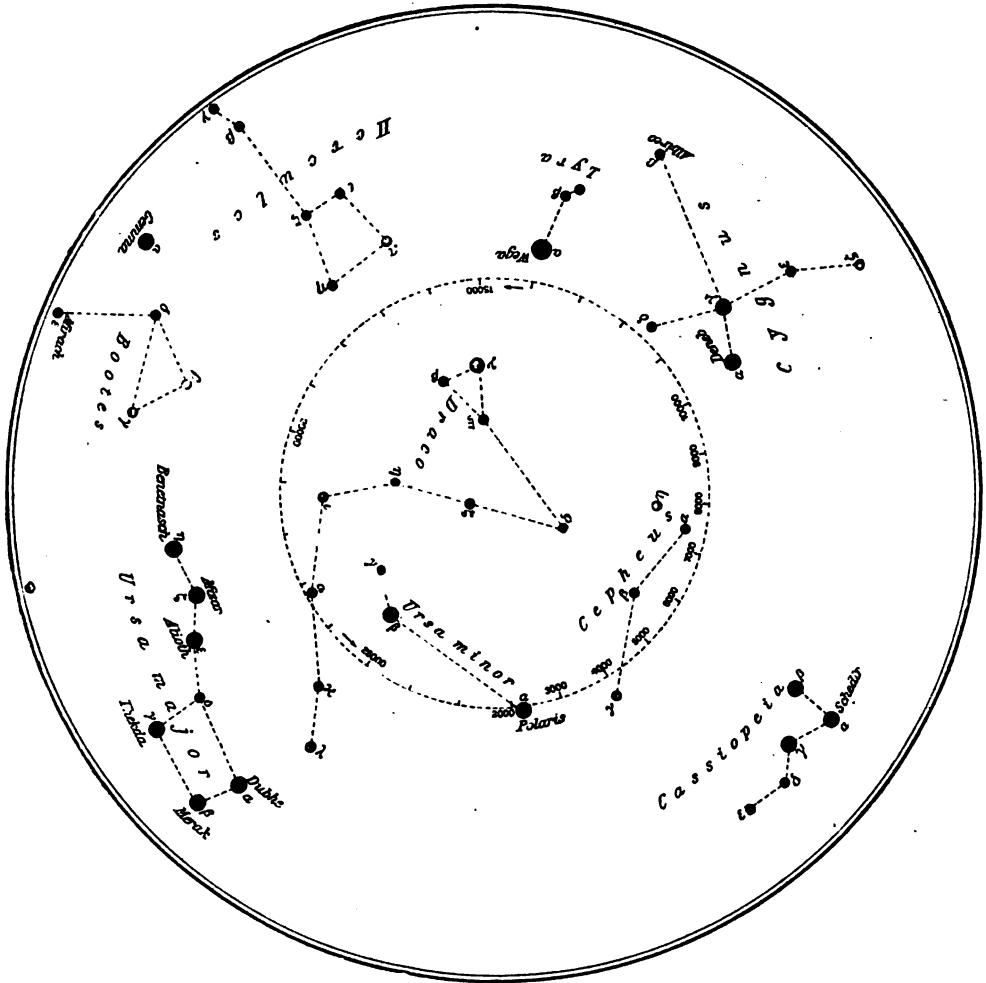
Движеніе небснаго полюса вокругъ полюса эклиптики вслѣдствіе прецессіи.
