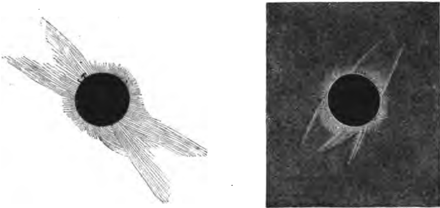
Старые рисунки солнечной короны, сдѣланные астрономами обсерваторіи Гарвардскаго Университета (Сѣв. Америка).
