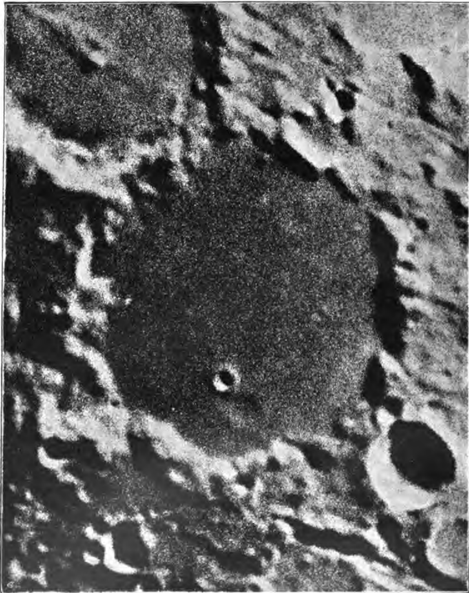
Циркъ Птоломей. По оригин. негативу Лихской обсерватори 10 ноября 1892 г. увеличенъ въ 16 разъ Л. Вейн-комъ въ Прагѣ.
