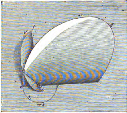
Положенія орбитъ земли, кометы Біелы и кометы Энке: а, b, c) орбита земли, а, e, g) орбита кометы Біелы, d, e, f) орбита кометы Энке. См. текстъ, стр. 235.
