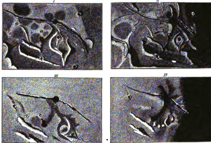
Новый кратеръ Клейна, Гигинусъ N. По рисункамъ Нейсона.
