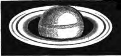
Сатурнъ съ карандашной линіей. Рис. Энке въ Берлинѣ 10 марта 1838 г.
