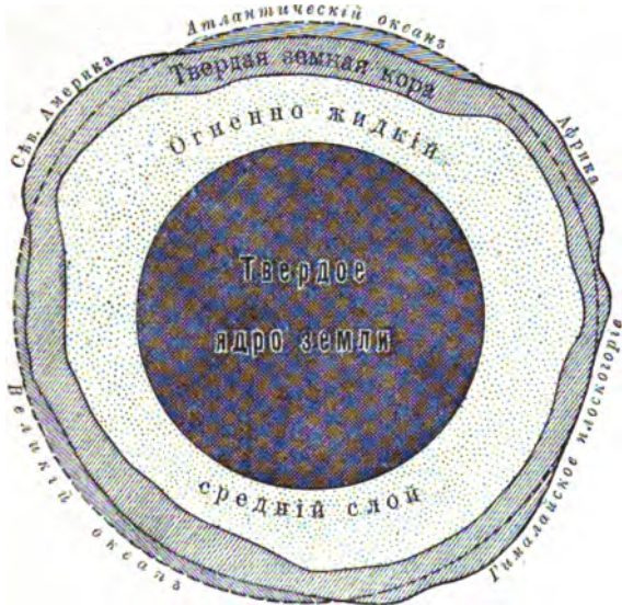
Поперечный разрѣзъ земли по параллельному кругу въ 30°, по Файю (отгосненія значительно преувеличены.)
