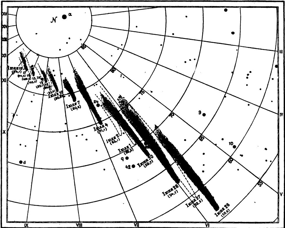
Видимое движеніе и измѣненіе длины хвоста большой кометы 1881 г., по наблюденіямъ Терби въ Лёвенѣ и В. Мейера въ Женевѣ.
