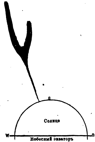
Кометоподобный объектъ, обнаруженный Гольденомъ на фотографическомъ снимкѣ, сдѣланномъ во время солнечнаго затменія 16-го апрѣля 1893 года.
