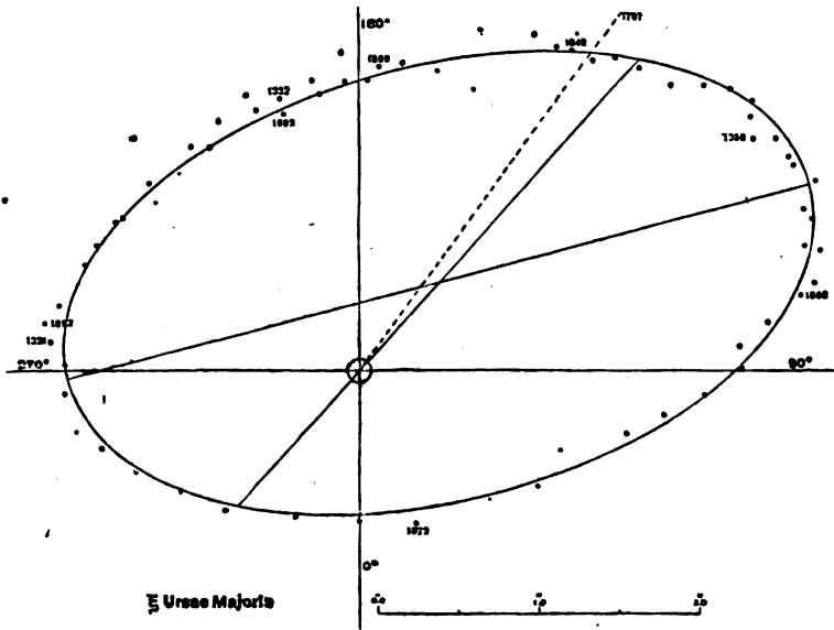
Орбита двойной звѣзды \xi Ursae majoris.
