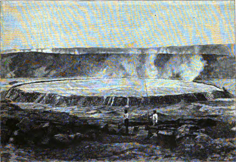
Вулканъ Килауеа съ Огненнымъ озеромъ на островѣ Гавайи. По фотографіи.
