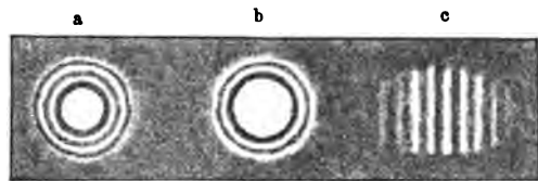
Явленія диффракціи.
