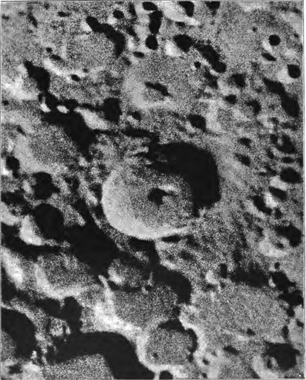
Лунный кратеръ Тихо съ его окрестностями. Увелич. въ 16 разъ Л. Вейнекомъ въ Прагѣ по оригиналу негативу Ликской обсерваторіи. Снимокъ сдѣланъ 10 ноября 1892 г.
