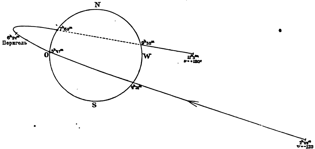
Видимое движеніе большой сентябрьской кометы 1882 г. вблизи ея перигелія. По Крейду. Ср. текстъ, стр. 217.
