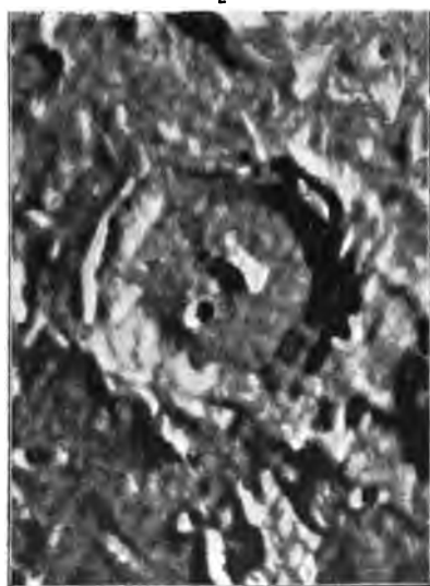
Лунный кратер Арзахель: 1) 15 августа 1888; 2) 27 августа 1888. Рисовано по 10-кратному увеличенію оригинальнаго негатива Ликской обсерваторіи Л. Вейнекомъ въ Прагѣ.
