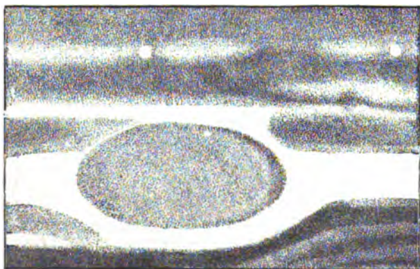
Красное пятно на Юпитерѣ: 1) 9 января 1895 г. рис., Гордона въ Патерсонѣ, Сѣв. Ам.; 2) 1880 г. рис. М. В. Мейера въ Женевѣ; 3) 20 октября 1893 г., рис. Антониади на обсерваторіи Фламмаріона въ Juvigny близъ Парижа; 4) 1889 г., рис. Килера на Ликской обсерваторіи; 5) съ полосой облаковъ, рис. 1886 г. Юнга; 6) 5 сентября 1888 г., рис. по увеличенію въ 630 разъ въ большой рефракторъ Ликской обсерваторіи; 7) 1878 г., рис. Нистена въ Брюсселѣ.
