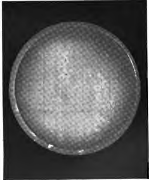
Фотографическій снимокъ Солнца съ факелами и хромосферою, Георга Хэля въ Чикаго.
