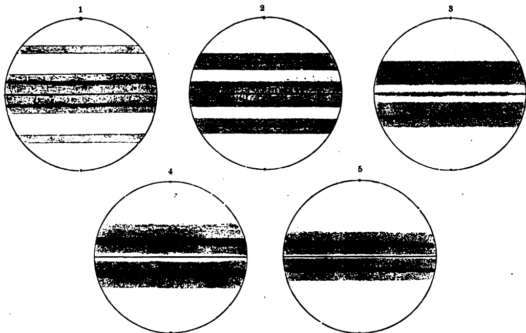
Распределёніе солнечныхъ пятенъ: 1) незадолго до минимума, 2) вскорѣ послѣ минимума, 3) передъ максимумомъ, 4) во время максимума, 5) послѣ максимума. См. стр. 295.
