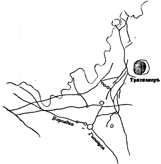
Борозда Гигинусъ и система бороздъ Трискеръ, представленныя схематически.
