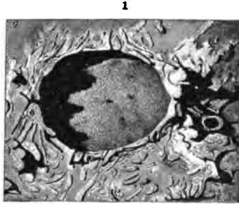
Циркъ Платонъ: 1) При восходѣ солнца, 2) при полуденномъ освѣщеніи. По Нейсову.
