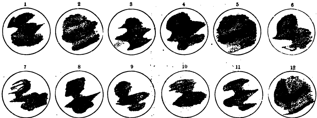
Рисунки третьяго спутника Юпитера, сдѣланные Шеберле и Кемпбелемъ въ Ликской обсерваторіи въ сентябрѣ и октябрѣ 1891 г.
