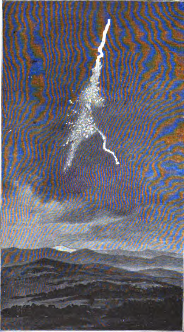
Метеоръ, видѣнный 27 июля 1894 года надъ Калифорніей. См. текстъ стр. 241 и 250.
