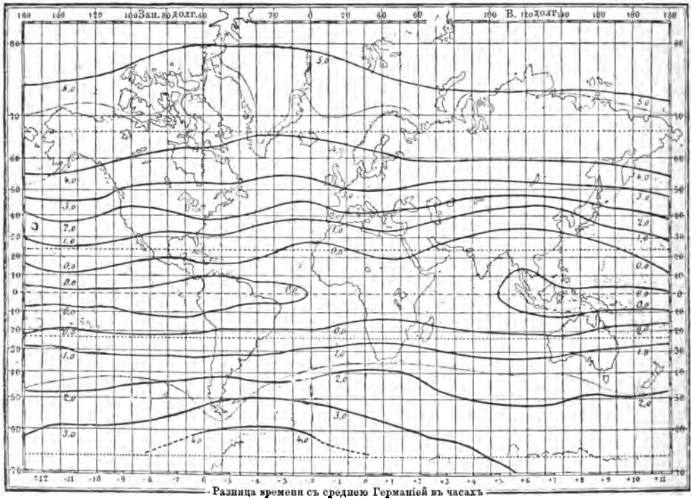
Линіи, соединяющія мѣста съ одинаковымъ напряженіемъ силы тяжести, опредѣляемымъ изъ наблюденій надъ качаніями маятника.
