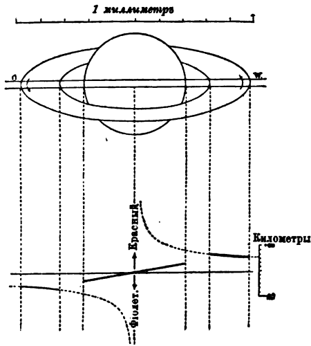
Положеніе линій поглощенія въ спектрѣ Сатурна и его колець, выведенное теоретически.
