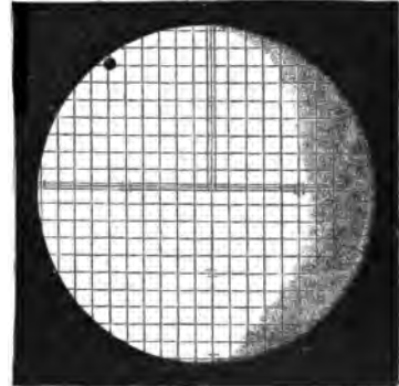
1) Венера на солнечномъ дискѣ, по фотогр., полученной въ Испани (вост. долг. отъ Берлина 2ч 33м 5с, сѣв. шир. 32° 38') въ 1874 г. 8 декабря, въ 6ч 31м 25с утра по ср. берл. времени. 2) Венера на солнечномъ дискѣ, по фотогр., полученной на ст. Аулендъ (вост. долг. отъ Берлина 10ч 11м 15с, южн. шир. 50° 32'), въ 1874 г. 9 декабря въ 6ч 33м 8с утра, по ср. берл. времени.
