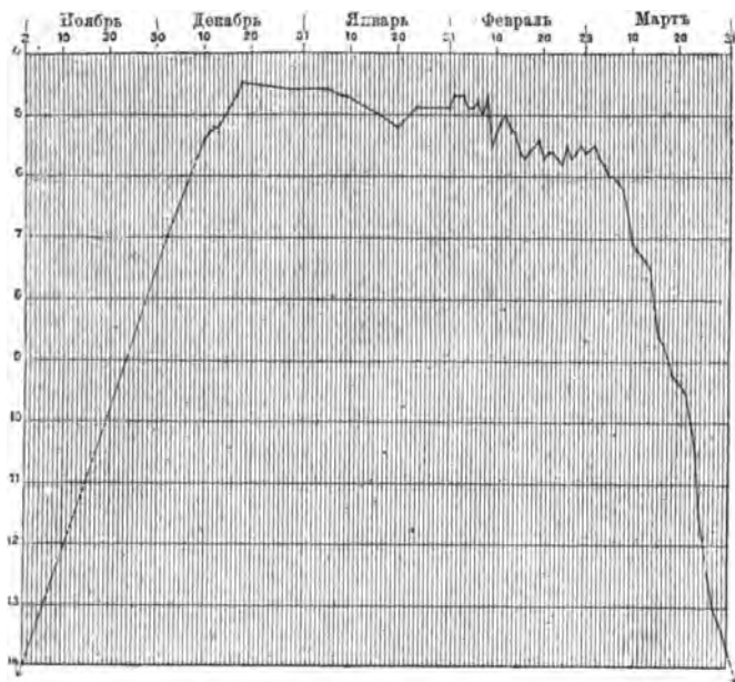
Кривая изменения блеска новой звѣзды въ Возничемъ 1891/92 г., по Фламариону
