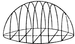
Видимыя пути свѣтилъ на земномъ экваторѣ.
