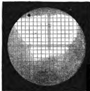
1) Венера на солнечномъ дискѣ, по фотогр., полученной въ Испани (вост. долг. отъ Берлина 2ч 33м 5с, сѣв. шир. 32° 38') въ 1874 г. 8 декабря, въ 6ч 31м 25с утра по ср. берл. времени. 2) Венера на солнечномъ дискѣ, по фотогр., полученной на ст. Аулендъ (вост. долг. отъ Берлина 10ч 11м 15с, южн. шир. 50° 32'), въ 1874 г. 9 декабря въ 6ч 33м 8с утра, по ср. берл. времени.
