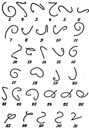
Различныя проэція проволоочной спирали (геликалы). По Хольдену.
