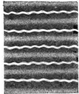
Летучія тѣни при солнечныхъ затменіяхъ. По П. Фаура.
