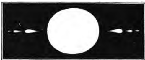
Предполагаемая форма поперечнаго сѣченія колець Сатурна представлена схематически и сильно преувеличена.
