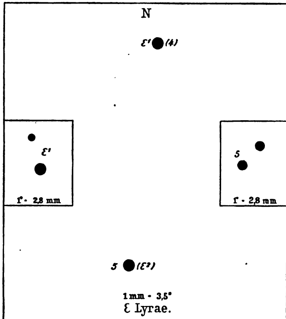
Четверная звѣзда \epsilon Лугае. Ср. текстъ, стр. 391.
