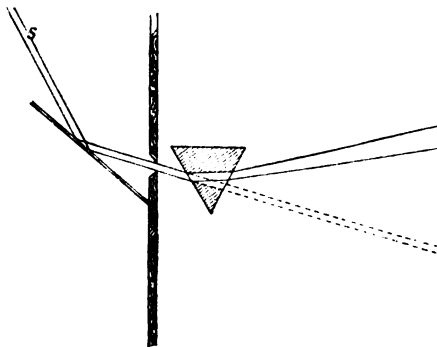
Дисперсія (свѣторазсѣяніе) бѣлаго свѣта въ призмѣ.
