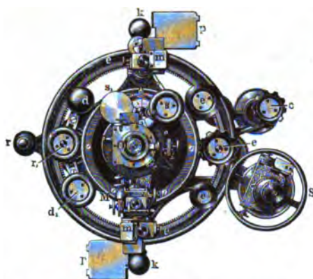
Окулярный конец трубы гелиометра.
